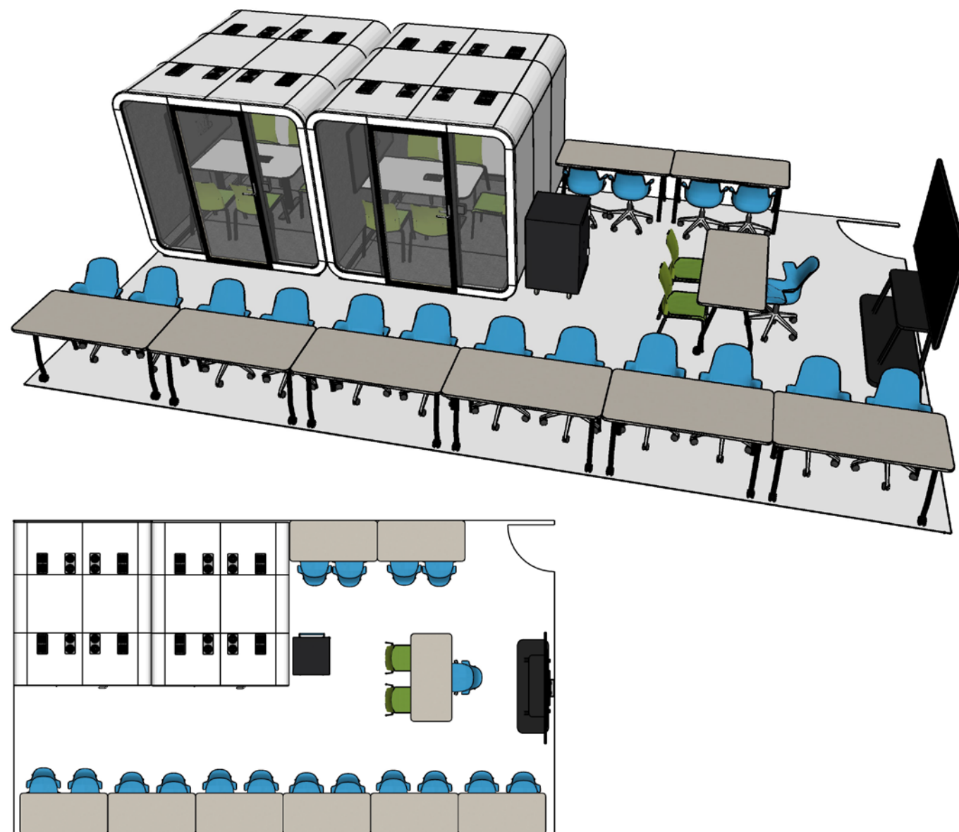
Fig 1. 3D CTE Área Total = 45m2
